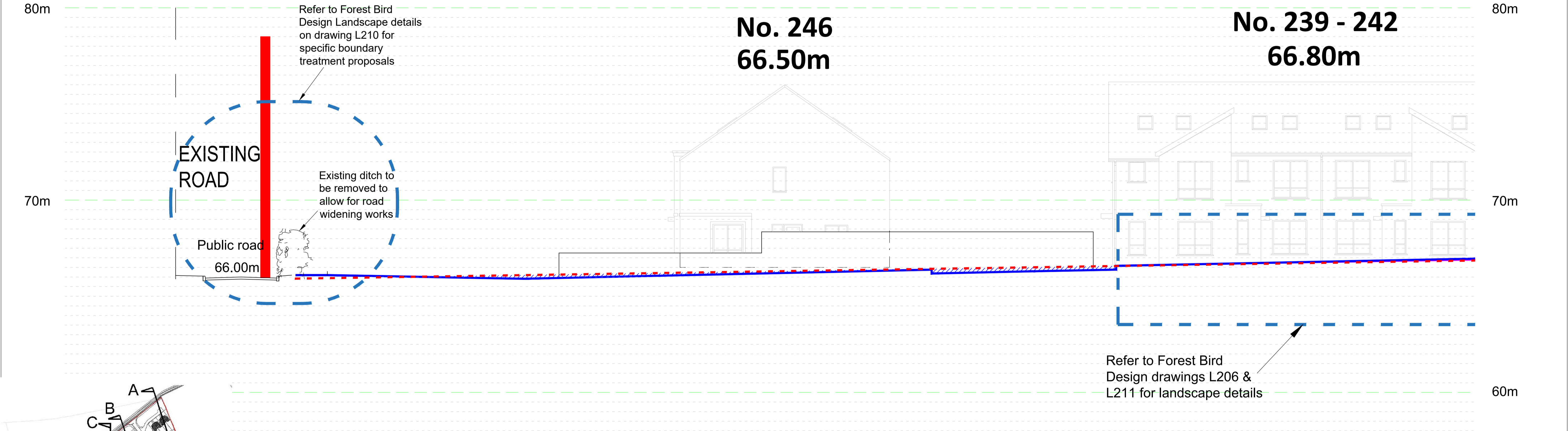
SITE SECTION G-G (part 1) Scale 1 : 100
