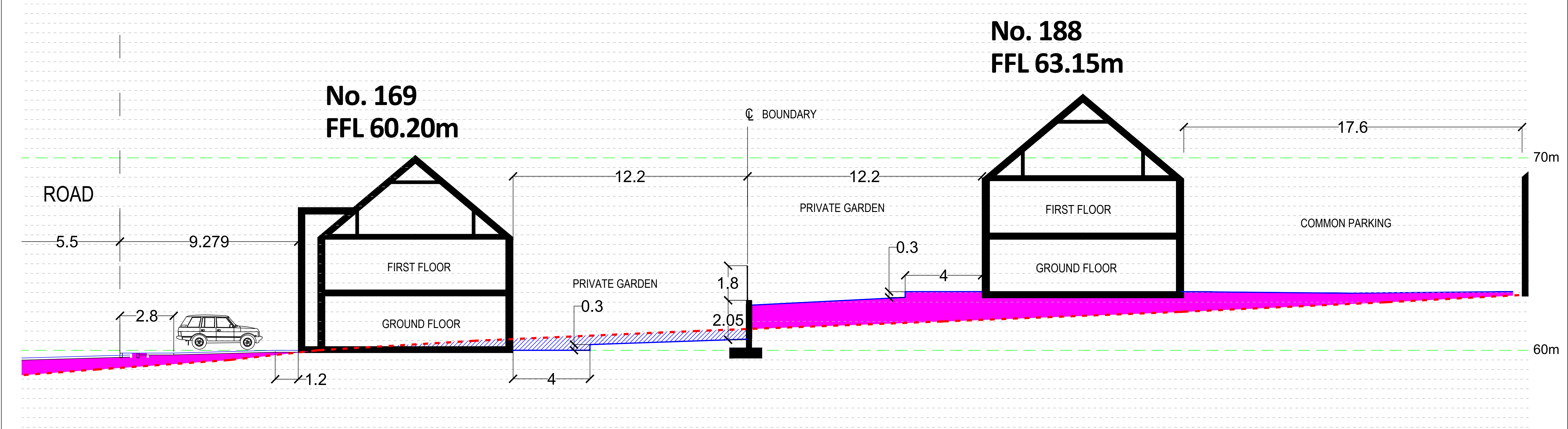
SITE SECTION A-A (part 4) Scale 1 : 100
