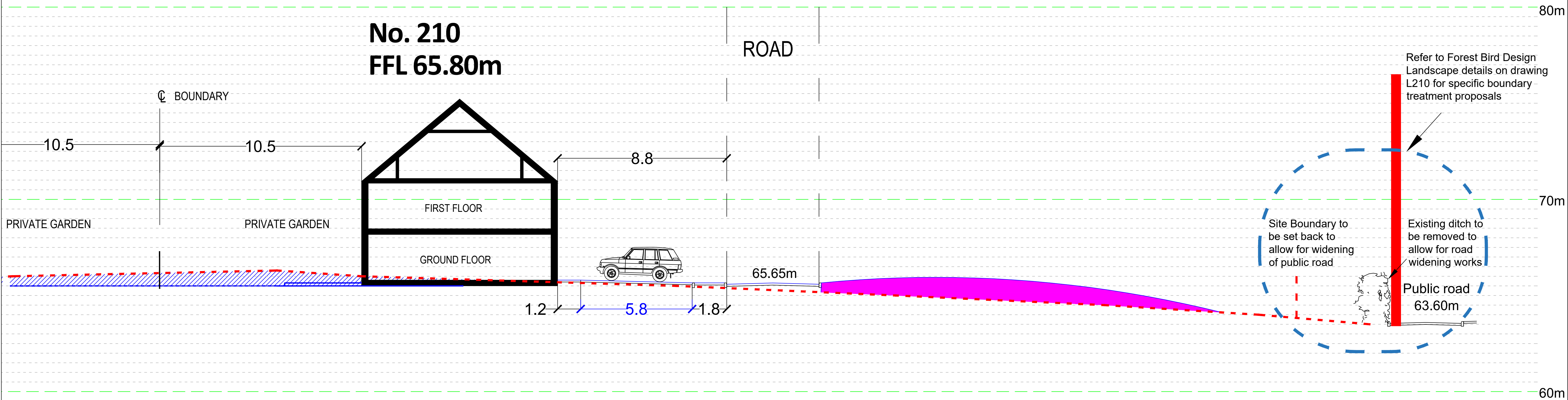
SITE SECTION A-A (part 6) Scale 1 : 100
