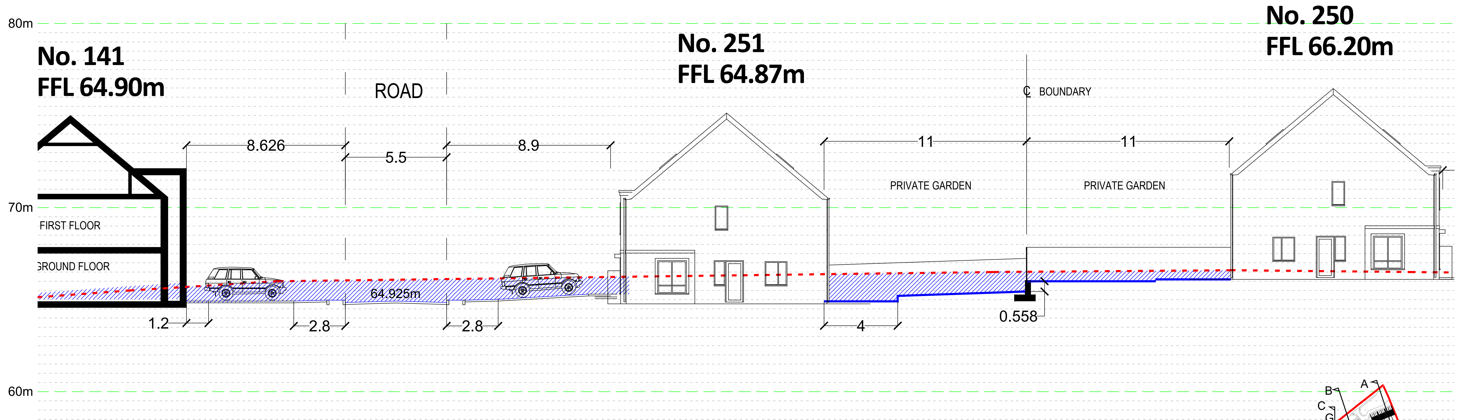
SITE SECTION C-C (part 4) Scale 1 : 100
