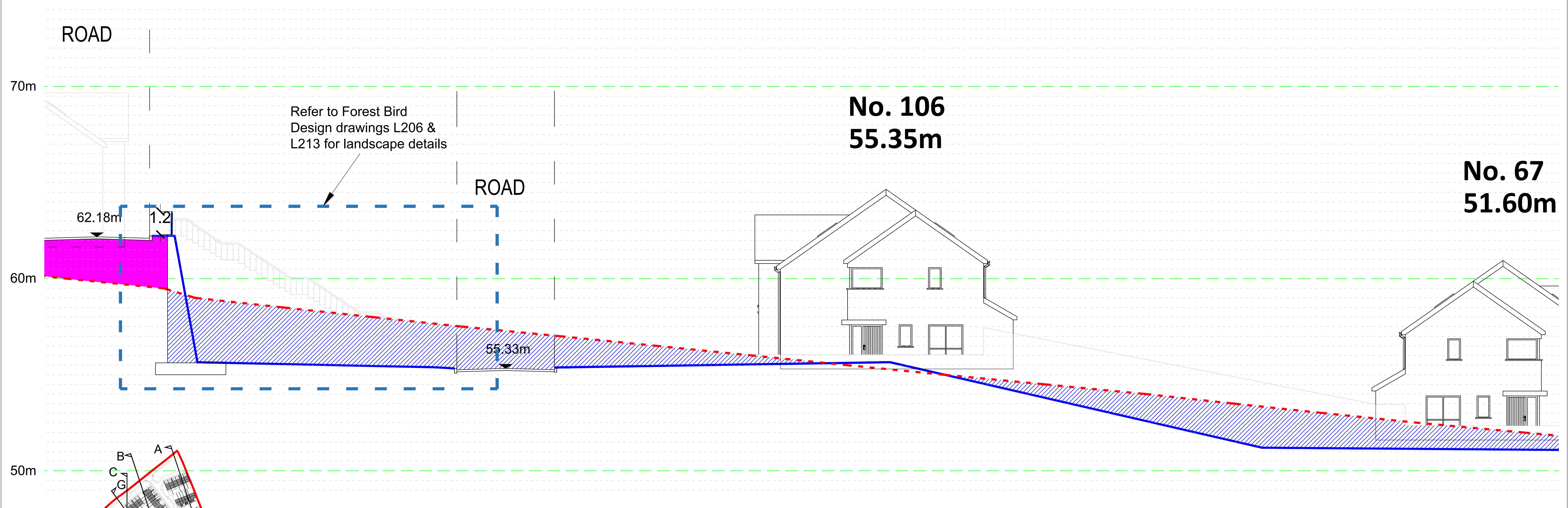
SITE SECTION G-G (part 4) Scale 1 : 100
